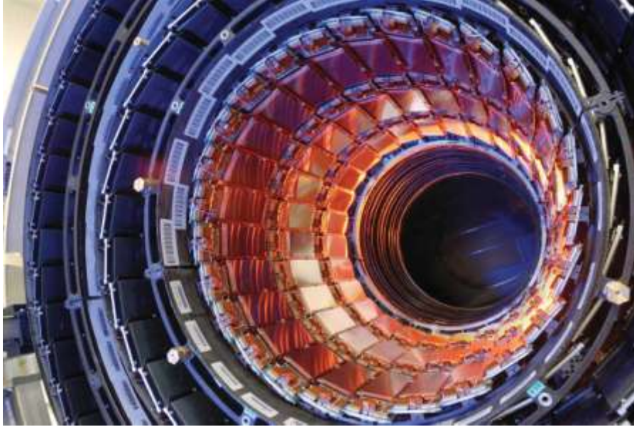
CERN Vortex
